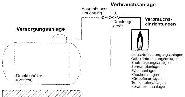
Bild 3: Verbrauchsanlage
